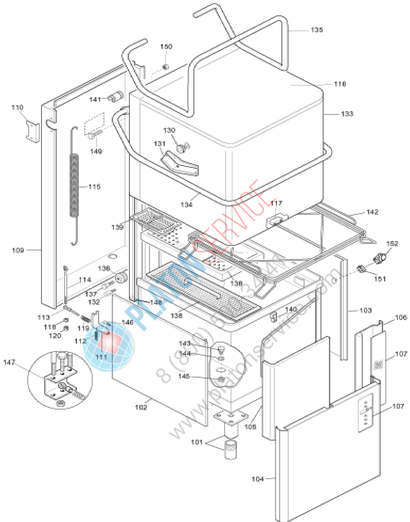
iLL 641804p1 Vista generale / Main view
